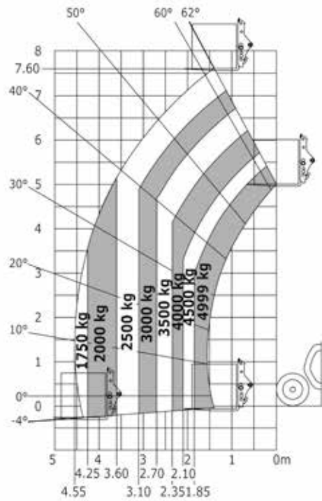
Диаграмма нагрузки для внедорожья (EN 1459 B) центр тяжести груза 500 мм
